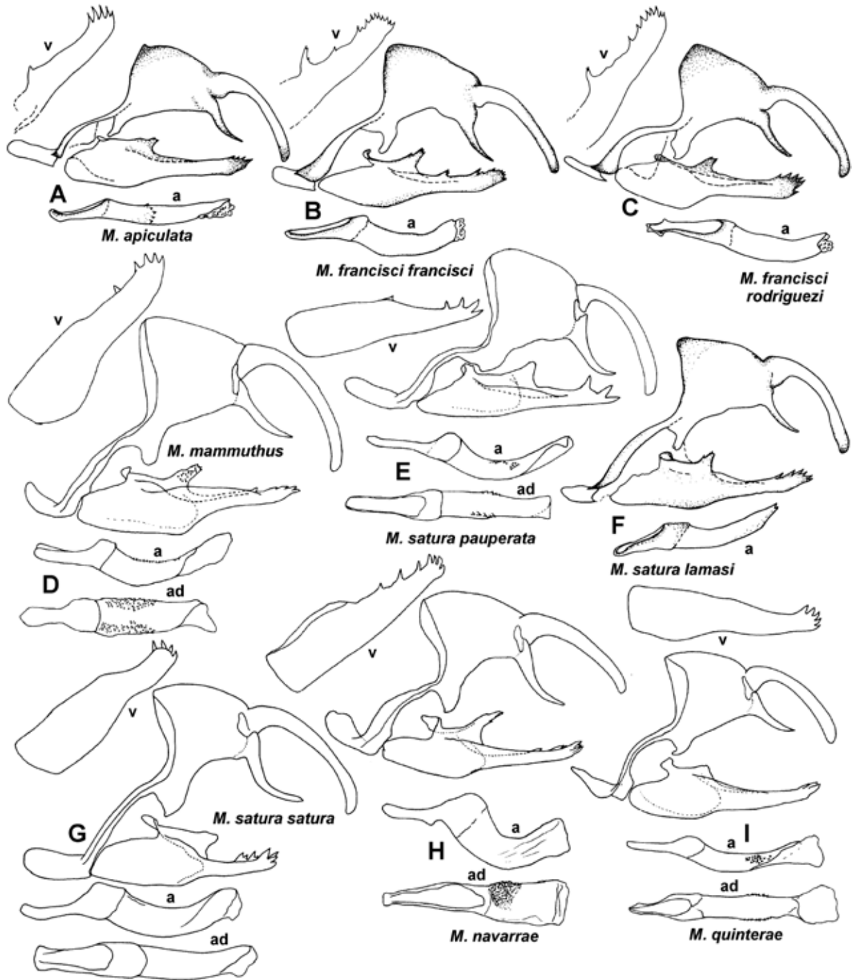
Fig. 11. Manerebia male genitalia, lateral view; v = valva ventral view, a = aedeagus lateral view, ad = aedeagus dorsal view. M. apiculata , M. francisci , M. mammoth n. sp., M. satura , M. navarrae , M. quinterae . See Appendix 5 for specimen data.
