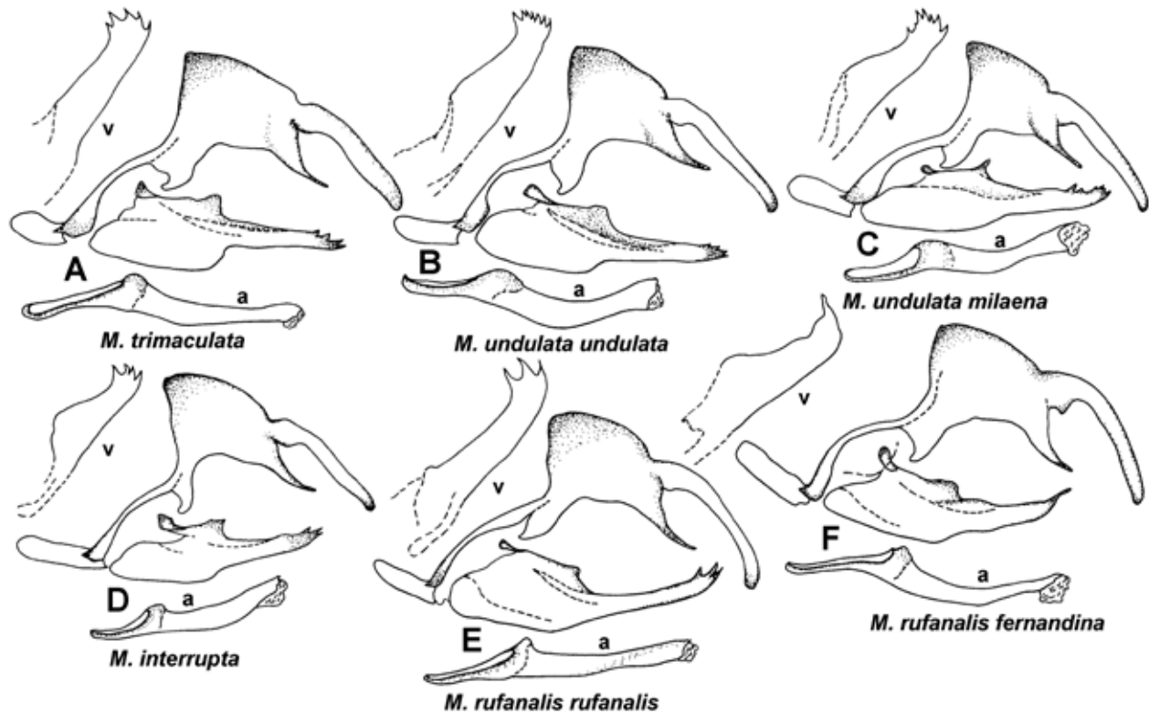
Fig. 13. Manerebia male genitalia, lateral view; v = valva ventral view, a = aedeagus lateral view, ad = aedeagus dorsal view. M. trimaculata , M. undulata n. sp., M. interrupta , M. rufanalis n. sp. See Appendix 5 for specimen data.
